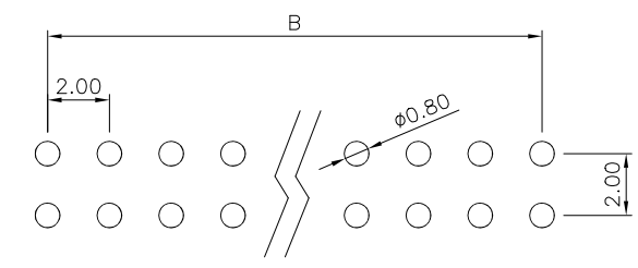
P.C.Board Layout
