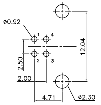
P.C.Board Layout
