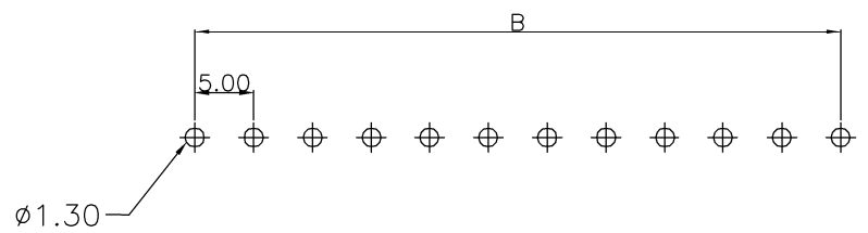
P.C.Board Layout
