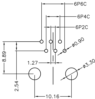
P.C.Board Layout
