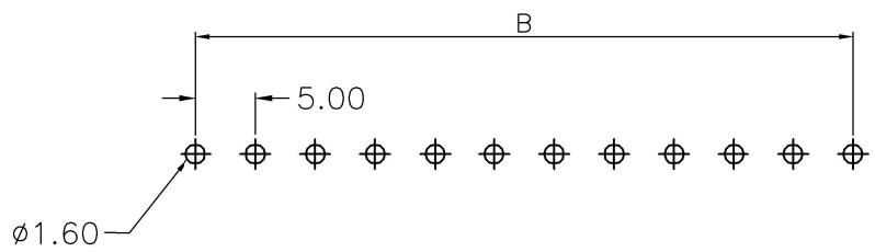
P.C.Board Layout
