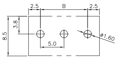
P.C.Board Layout
