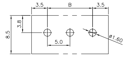
P.C.Board Layout
