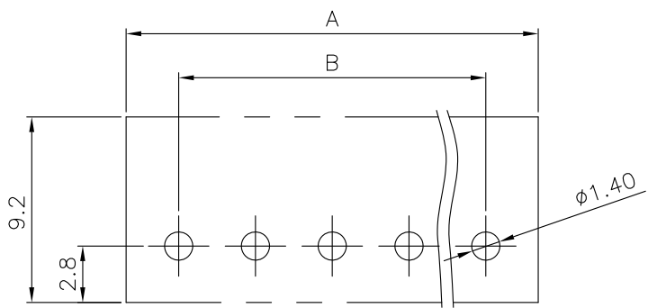
P.C.Board Layout
